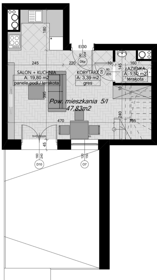
kondygnacja 1
