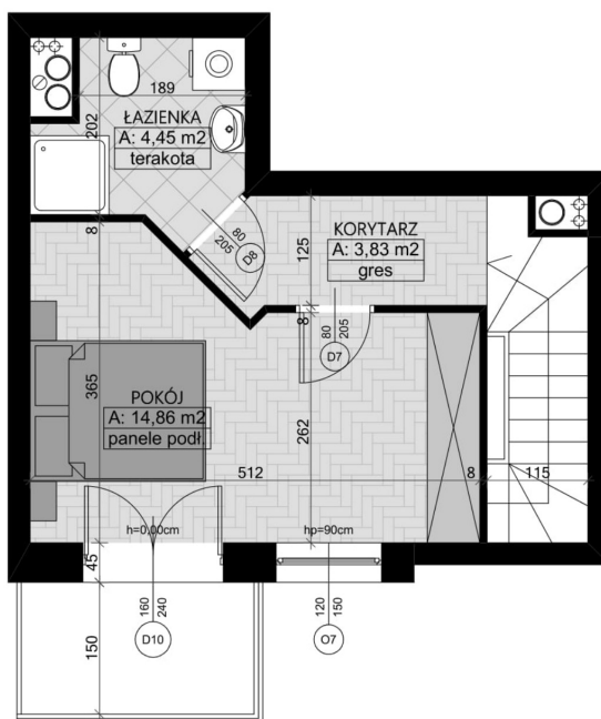
kondygnacja 2
