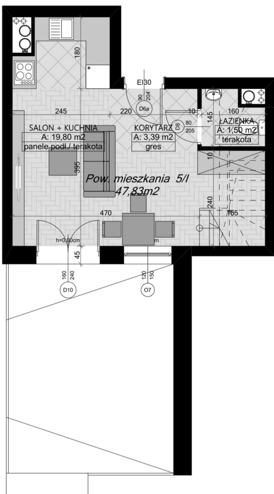
kondygnacja 1
