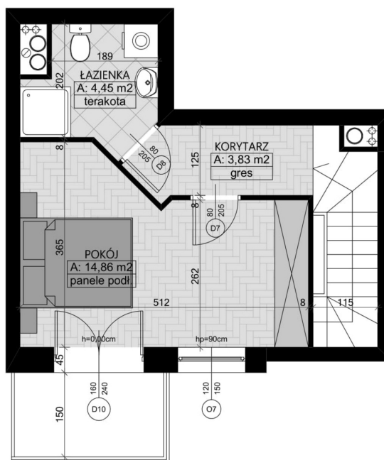
kondygnacja 2
